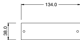
ブランクパネル (塩ビシート) 詳細図
