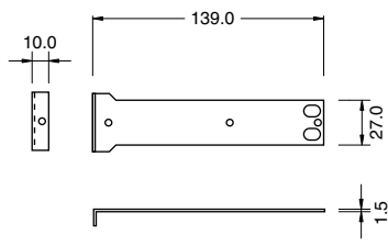
Vnet インターフェイスL字取付金具 詳細図
