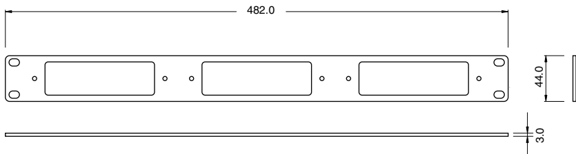
本体 詳細図
