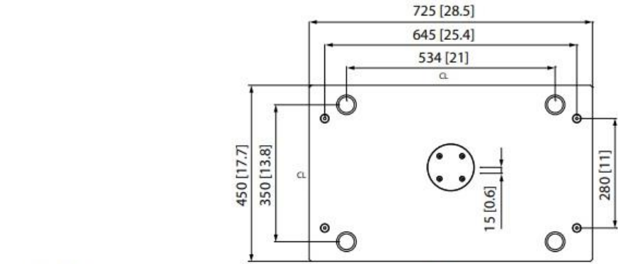
TOP
