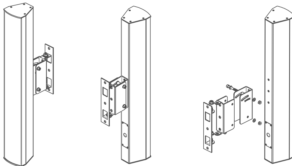
パンチルト ブラケット(UBX8接続時)
