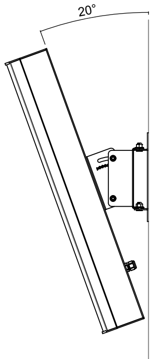
パンチルトブラケット使用時の垂直調整角度
