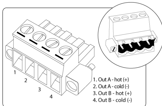
4ピンユーロブロックコネクター リモート
