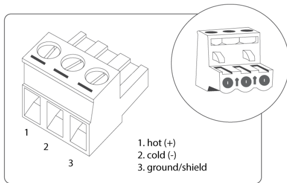
3ピンユーロブロックコネクター リモート
